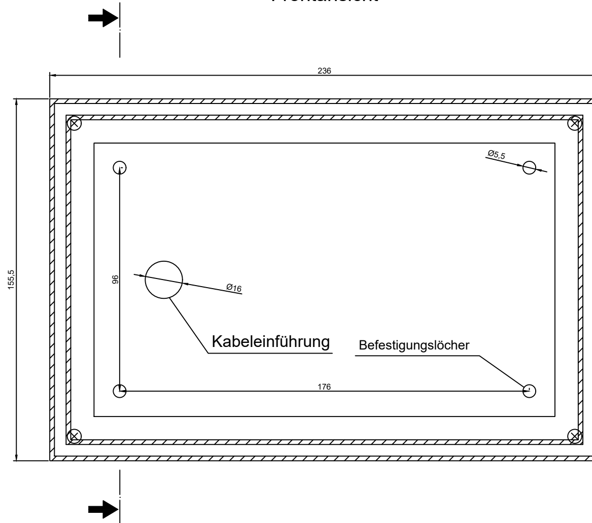
Frontansicht
